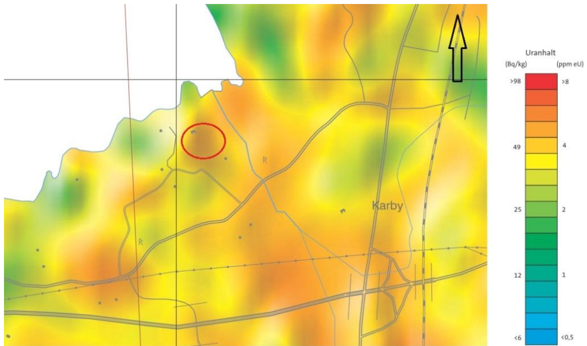
Figur 8. Utdrag ur SGUs flyggeofysiska karta – Uran. Aktuellt område markeras med röd cirkel. (källa: http://apps.sgu.se/kartgenerator ).
