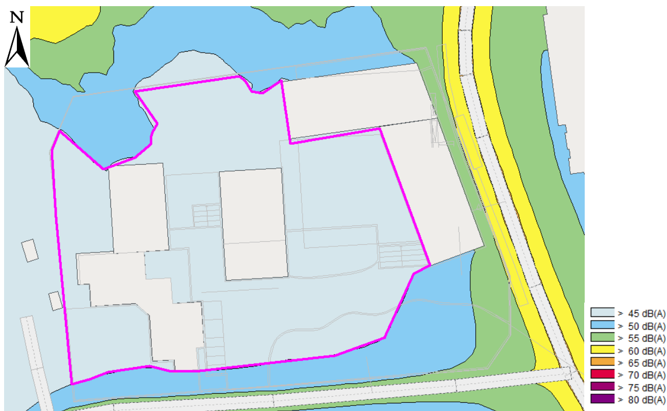
Figur 9. Ekvivalent ljudnivå på 1,5 m höjd. Inom hela den rosamarkerade ytan kan uteplatser som klarar riktvärde med avseende på både ekvivalent och maximal ljudnivå förläggas.
