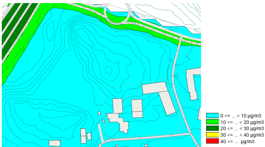
Figur 12. NO 2 årsmedelvärde för prognos
