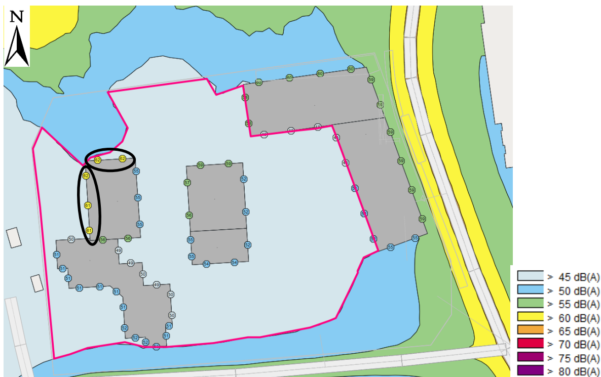
Figur 5. Ekvivalent ljudnivå inom planområdet. Riktvärdet 60 dBA ekvivalent ljudnivå överskrids för byggnaden inringad i rött.
