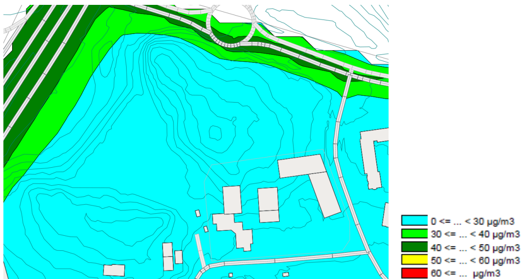
Figur 13 NO 2 dygnsmedelvärde för nuläge
