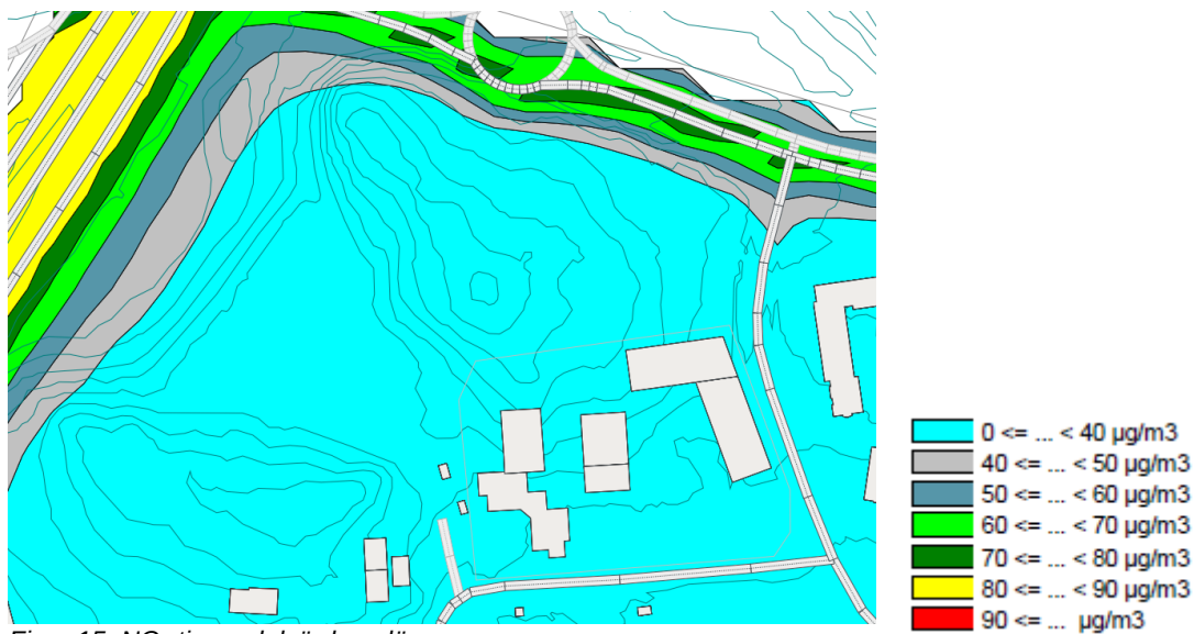
Figur 15. NO 2 timmedelvärde nuläge
