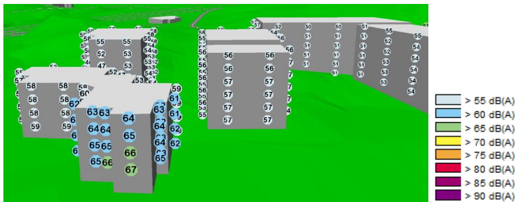
Figur 7. Maximal ljudnivå vid fasad, vy från Näsby Allé mot norr.
