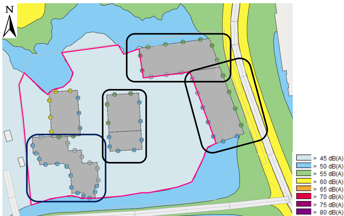
Figur 4. Ekvivalent ljudnivå vid fasad. Inringade byggnaders fasad klarar riktvärdet 60 dBA ekvivalent ljudnivå.
