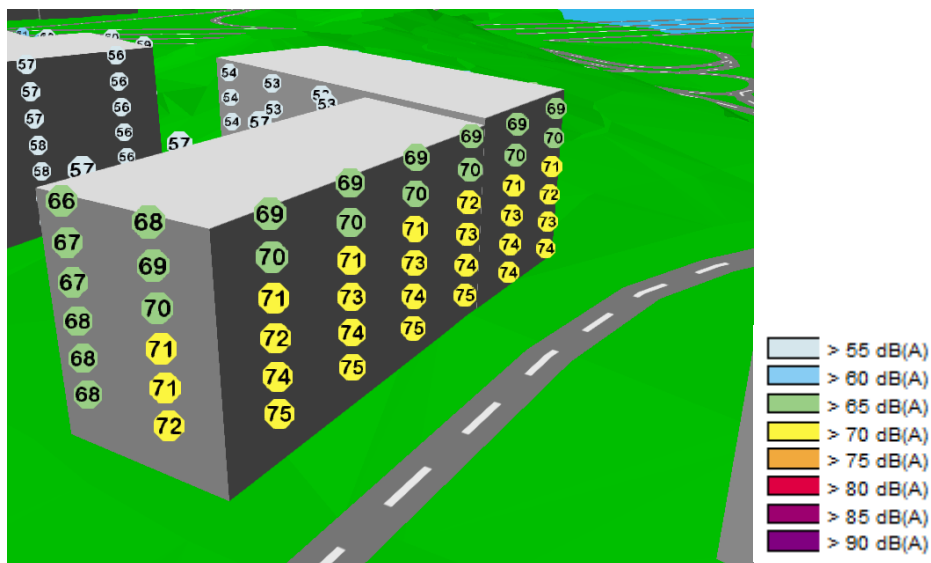
Figur 8. Maximal ljudnivå vid fasad för hus 5, vy från Herkulesvägen mot nordväst.
