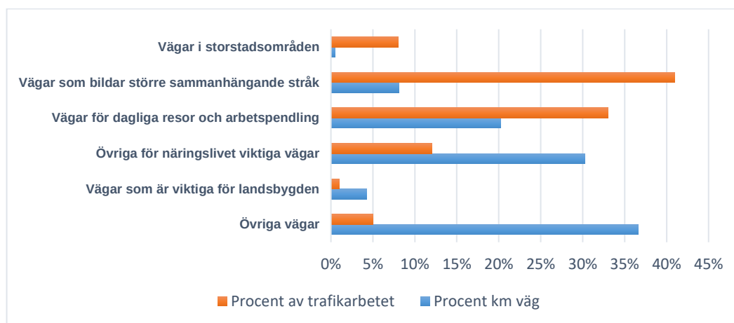
Figur 6. Vägsystemets indelning.
