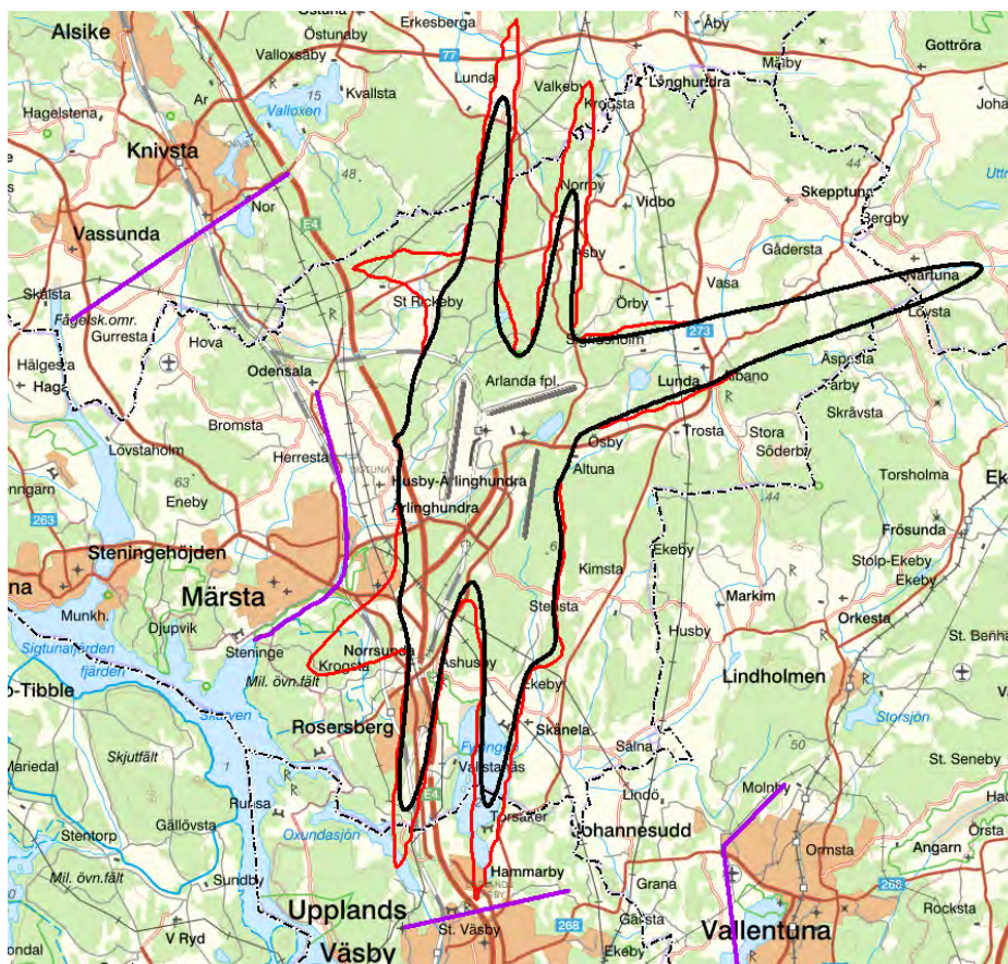
Karta 28. Utfall bullerpåverkan 2019. Svart linje FBN 55 dBA, röd linje maxbuller sammanslaget. Lila linjer är "NRL-linjerna", villkor 18-21 i miljötillståndet.
