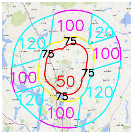
Karta 19. Procedurhinderytor gällande endast Arlanda, höjder anges i AMSL (RH2000).
