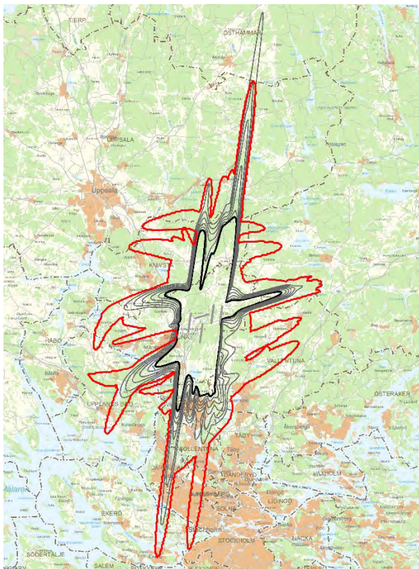
Karta 31. Flygbullerkurvor FBN 50-55 dB(A) samt maxbuller 65 dB(A).
