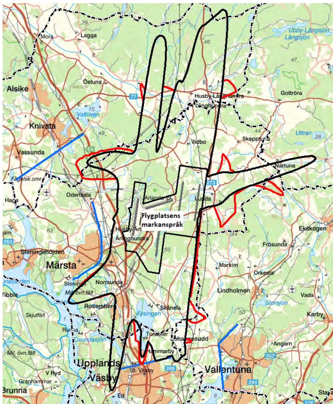
Karta 30. Flygbullerkurvor för ett framtidsscenario med 540 000 flygrörelser. Svart linje 55 dBA, röd linje maxbuller sammanslaget. Blå linjer är "NRL-linjerna", villkor 18-21 i miljötillståndet.
