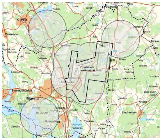
Karta 20. Skyddsområden för DME-anläggningar.
